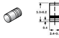
DL-41
