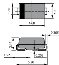
SMA (DO-214AC)
