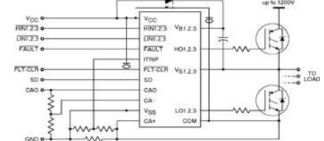
3-фазные драйверы с инверсией
