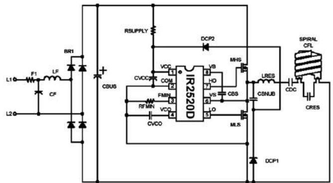
ТИПИЧНАЯ СХЕМА ПРИМЕНЕНИЯ
