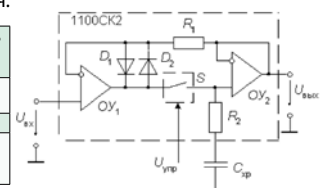
ПРИНЦИПАЛЬНАЯ СХЕМА
