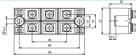
INT-A-Pak
