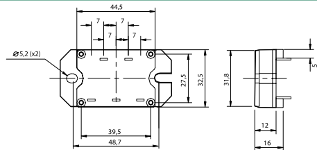
MTP-A
