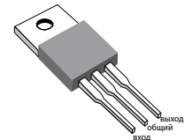
TO-220 (КТ-28) (для КР1158ххВ,Г)
