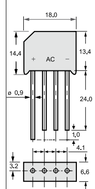
2KBB
