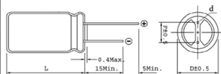
ГАБАРИТНЫЕ РАЗМЕРЫ D (MM) X L (MM)
