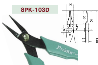
8PK-103D Круглогубцы (140 мм)
