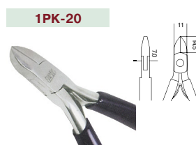
1PK-20 Бокорезы (115 мм)
