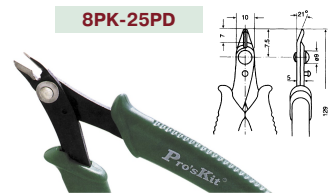
8PK-25PD Бокорезы для пров. до 1.3 мм 8PK-25PD-C Бокорезы с фиксатором
