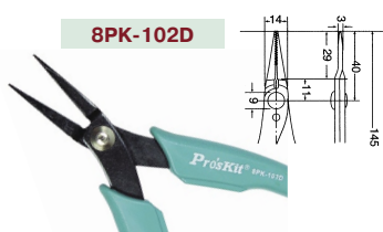
8PK-102D Удлиненные плоскогубцы (145 мм)
