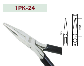
1PK-24 Тонкогубцы (125 мм)
