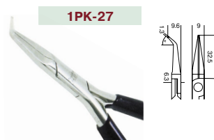
1PK-27 Тонкогубцы загнутые (135 мм)
