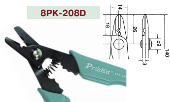
8PK-208D Кусачки Ø1.3 мм/стриппер Ø 0.4 мм (140 мм)
