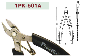
1PK-501A Миниатюрные бокорезы (90 мм)
