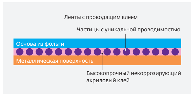
Рис.2. Поперечное сечение экранирующей ленты с проводящим клеем
